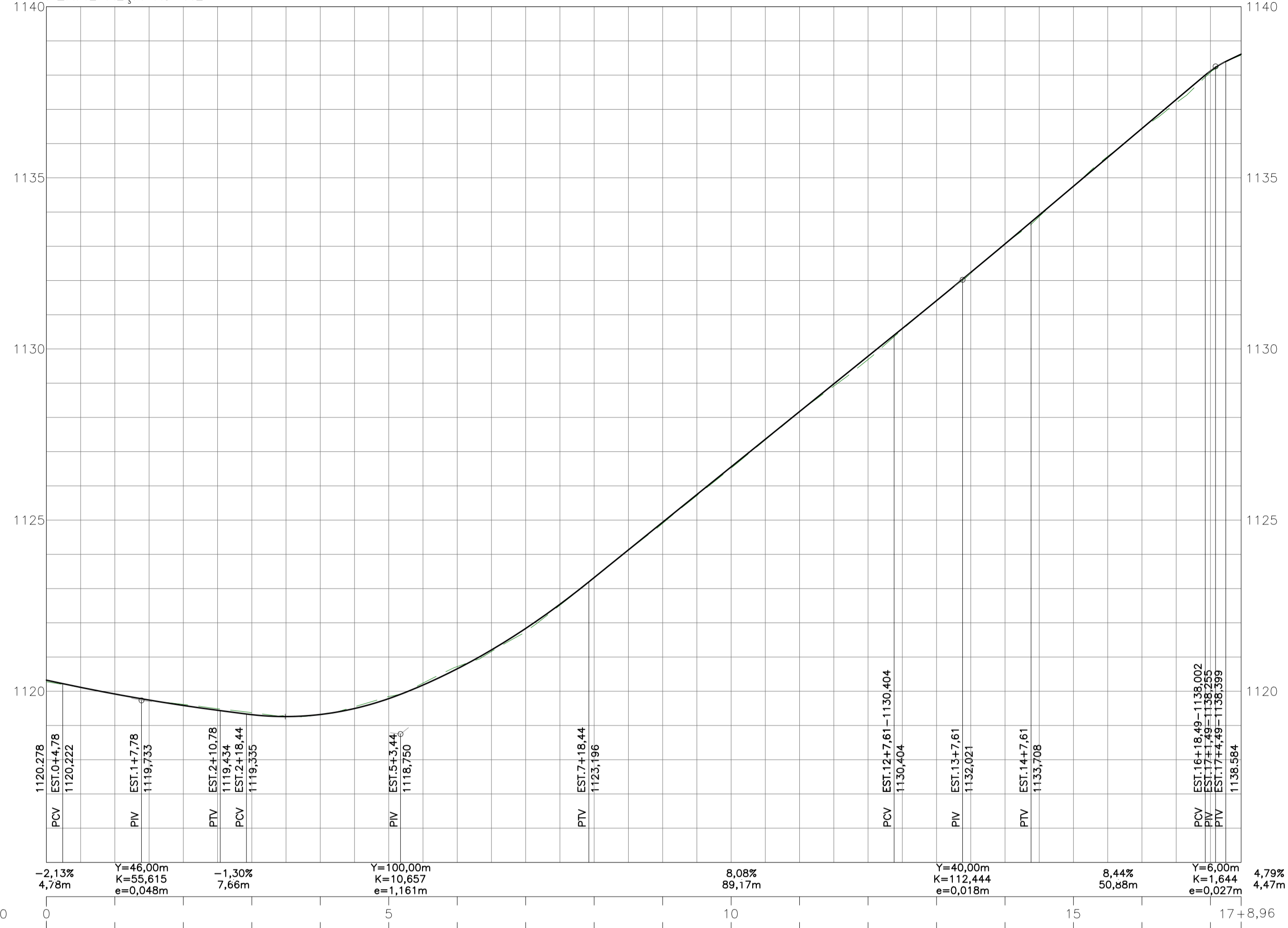
PERFIL ALÇA RJ-NL
