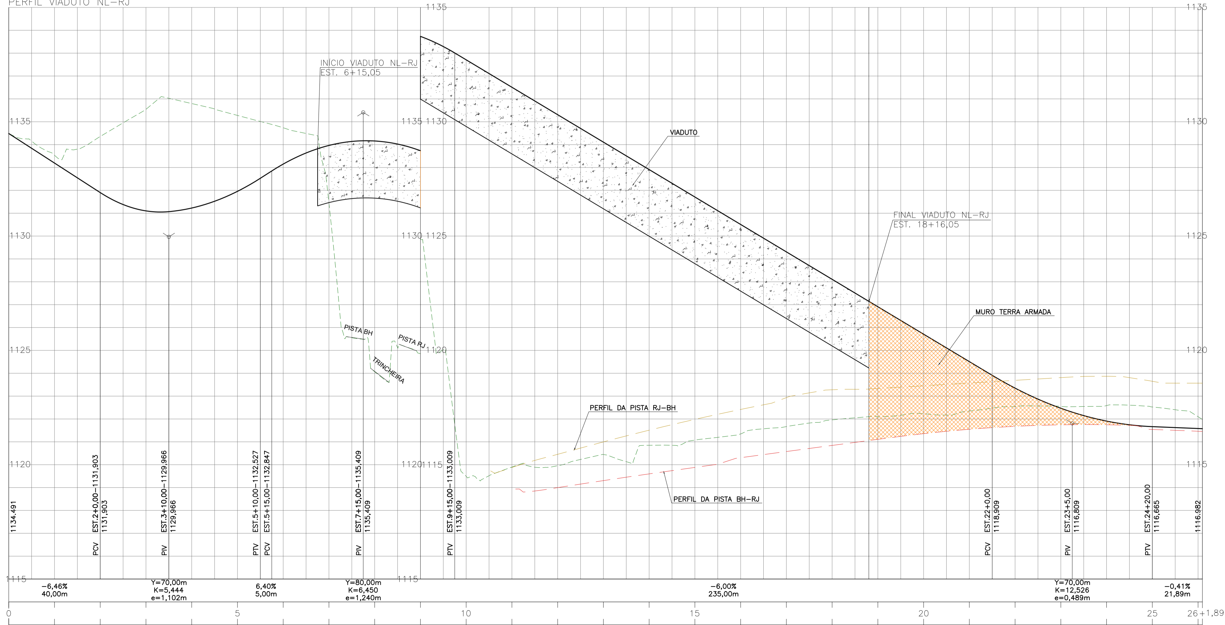
PERFIL VIADUTO NL-RJ
