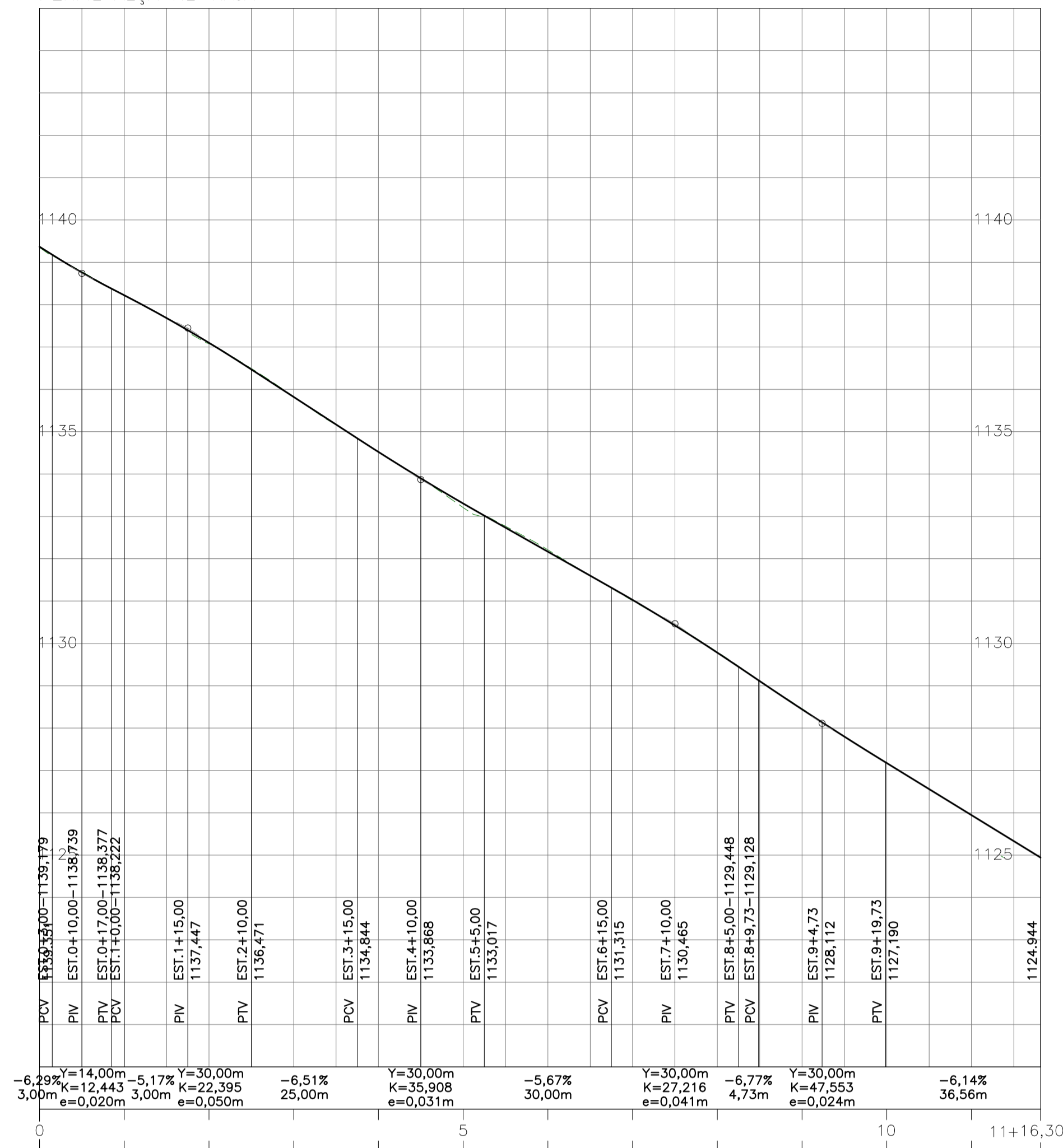
PERFIL ALÇA NL-RAJA
