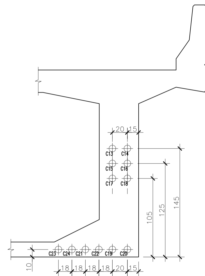
SEÇÃO 12 ESC. 1:25
