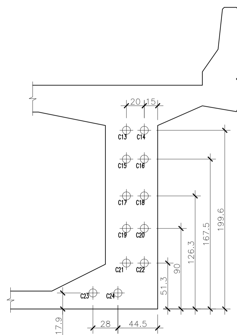
SEÇÃO 18 ESC. 1:25
