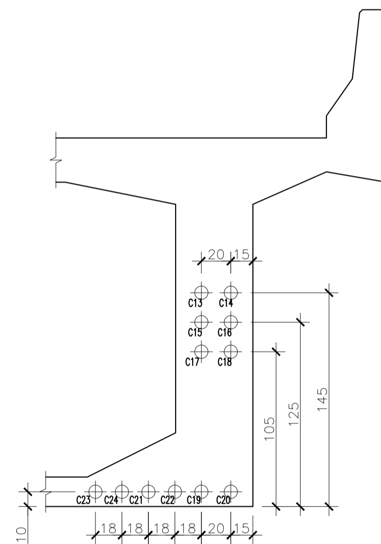
SEÇÃO 13 ESC. 1:25
