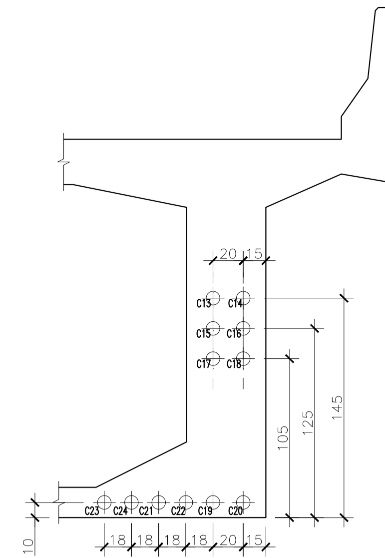
SEÇÃO 14 ESC. 1:25
