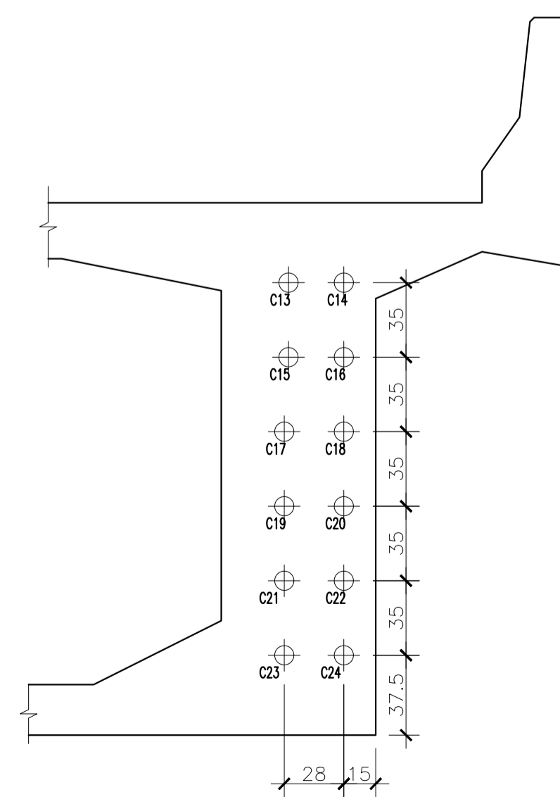
SEÇÃO 19 ESC. 1:25
