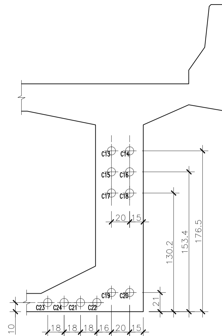
SEÇÃO 13 ESC. 1:25
