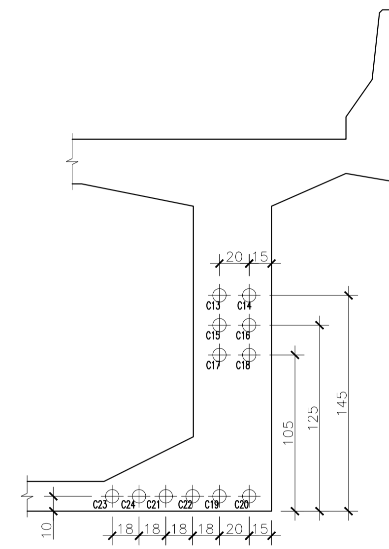
SEÇÃO 14 ESC. 1:25
