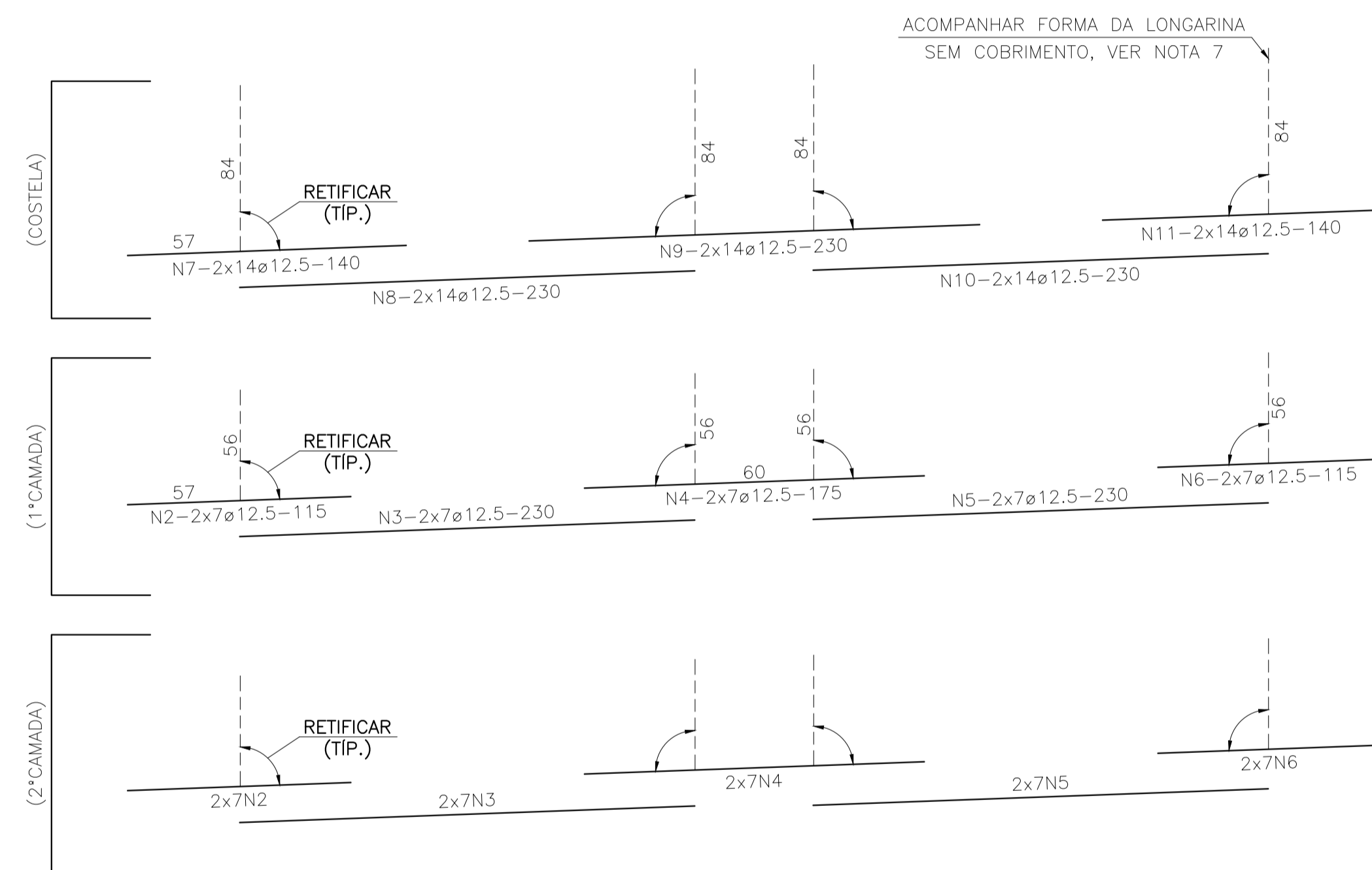
TRANSVERSINAS - ELEVÇÃO (12x) ESC.1:25
